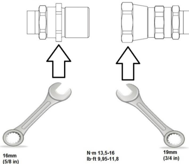
Kuva 9: Pikaliitäntätyyppi "X"
