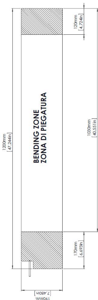
Figura 19: Zone di piegatura Evaporatore 1200x190
