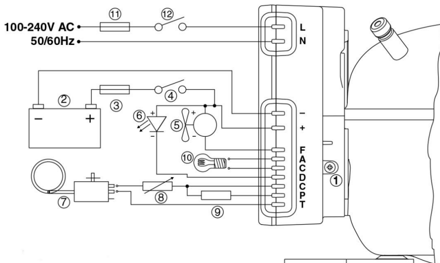
Sähkökaavio 12 Vdc - 24 Vdc - 100 Vac/240 Vac
