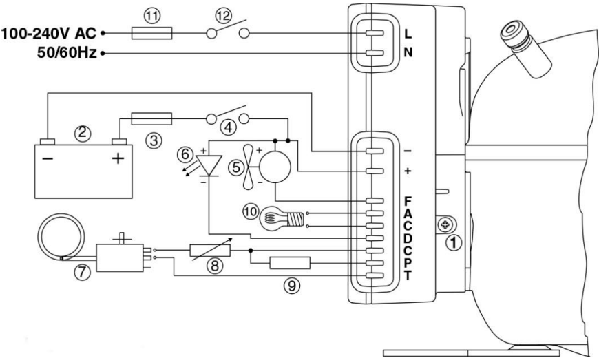
Esquema eléctrico 12Vdc-24Vdc - 100Vac/240Vac
