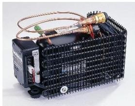
Lauhdutinyksikkö
