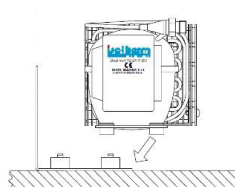
Instalación en mamparo horizontal
