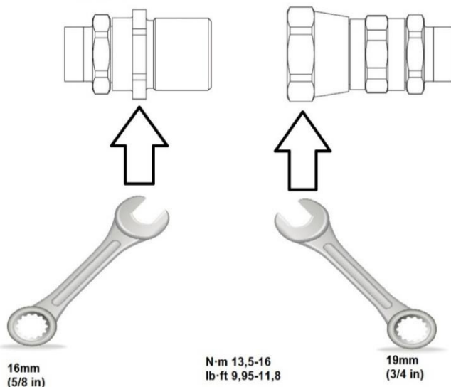
Afbeelding 9: "X"-vormige snelkoppeling
