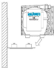
Installation an vertikaler Schottwand
