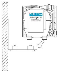
Installatie aan een verticale scheidingswand
