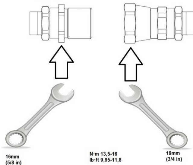
Рисунок 9: Категория быстросъемной муфты типа "О"
