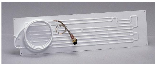
Evaporatore
